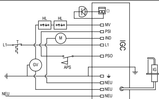
ELECTRICAL LADDER DIAGRAM/SCHEMA D'ÉCHELLE ÉLECTRIQUE/ DIAGRAMA ELÉCTRICO DE ESCALERA
